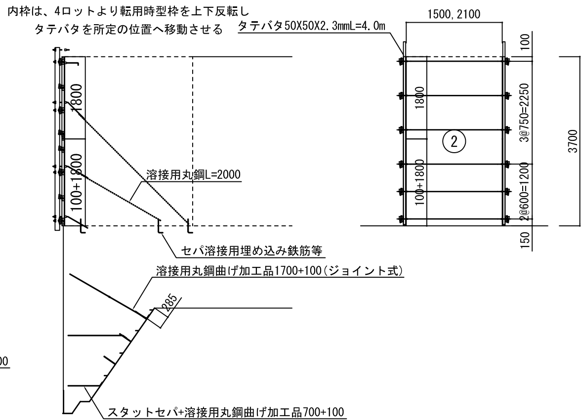
隔壁部断面図
