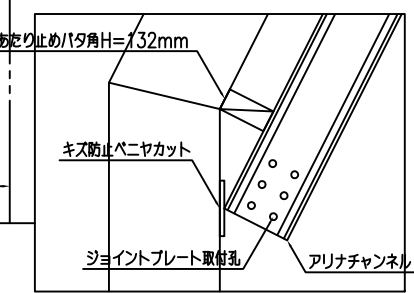
型枠下部詳細図
